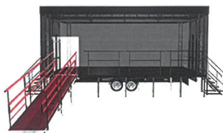
Rys. 3. Widok rozłożonej sceny mobilnej z rampą Źródło: Producent https://www.alspaw.com.pl/index.php/pl/produkty/sceny-mobilne/wyposazenie-dodatkowe z dnia 11.07.2024
